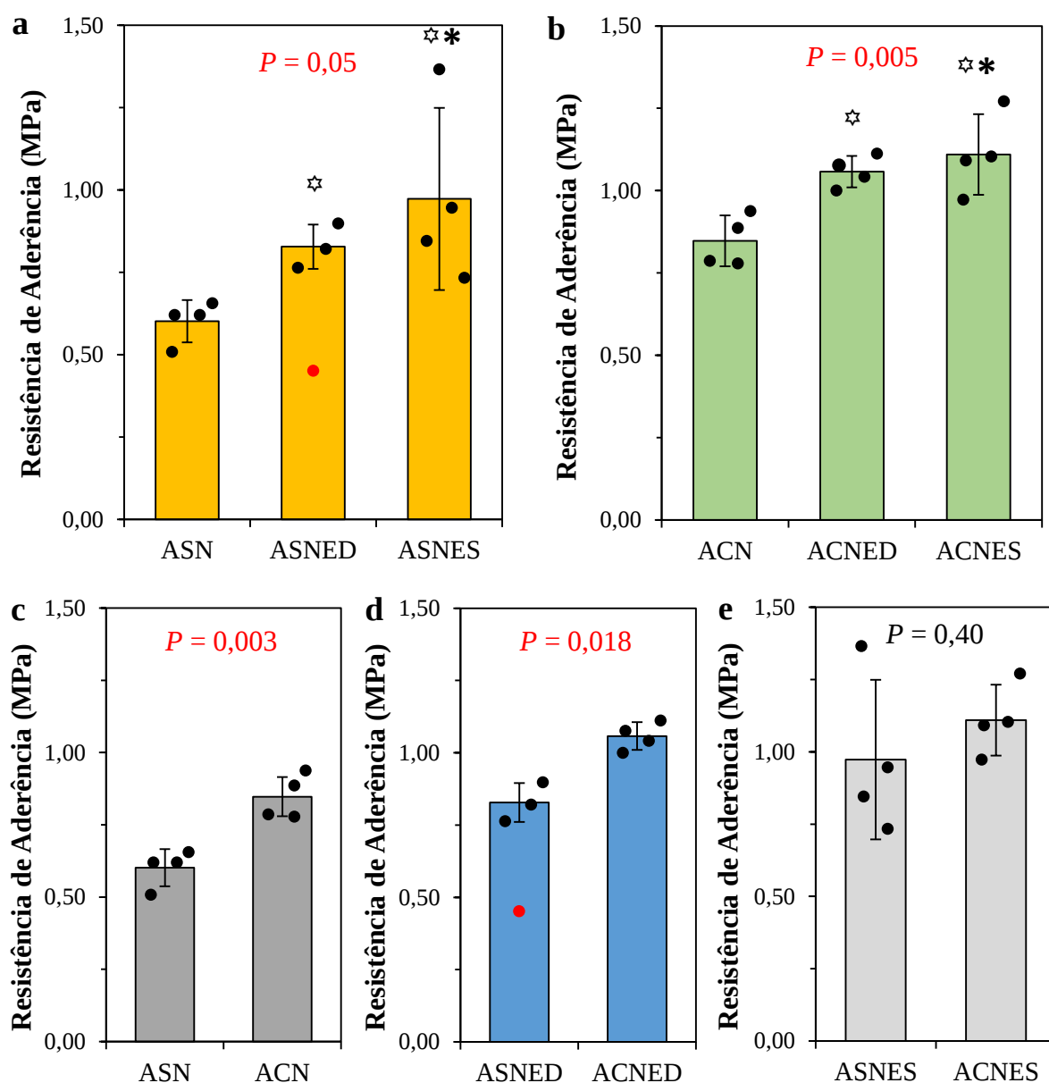
Figura 4.16 - Resultados de resistência de aderência bambu concreto aos 28 dias. (a) famílias sem nó; (b) famílias com nó; (c) famílias de referência; (d) famílias com espiral dupla; (e) famílias com espiral simples. ● valor discrepante. * P < 0,05 em relação à referência. ☆ P > 0,05 entre si. n=4 , variância significativa quando P < 0,05 . Teste t – Student e ANOVA, Tukey.
