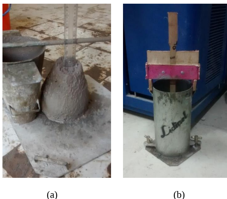
Figura 3.6 - Produção concreto. (a) Abatimento tronco de cone (b) Sistema de moldagem.
