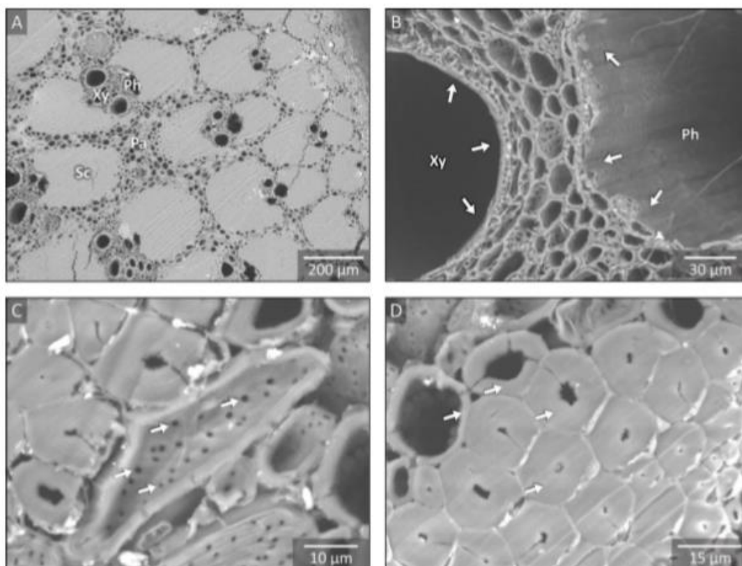
Figura 2.6 - Micrografias eletrônicas de varredura da seção transversal do bambu. (A) elementos dos feixes vasculares: xilema (Xy), floema (Ph), esclerênquima (Sc) e parênquima (Pa); (B) detalhe das paredes celulares do floema, dissolvida, e do xilema; (C) detalhe das pontoações celulares; (D) detalhe dos diferentes níveis de lignificação das paredes de células do esclerênquima. Fonte: Palombini (2016).
