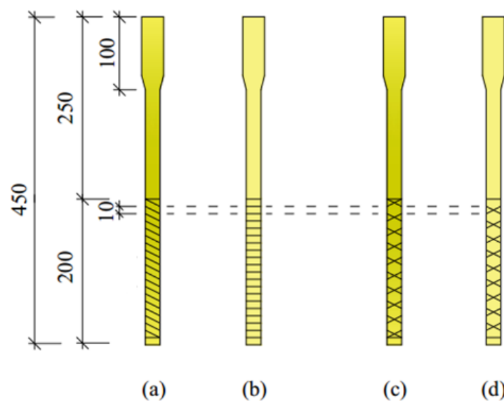
Figura 3.7 - Detalhamento do bambu sem nó para o ensaio de arrancamento.
