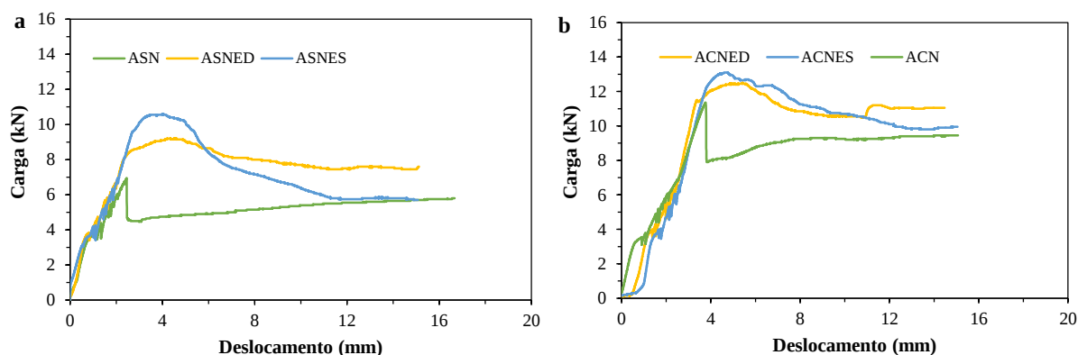
Figura 4.17 - Diagrama carga x deslocamento do ensaio de arrancamento bambu concreto. (a) famílias sem nó; (b) famílias com nó.
