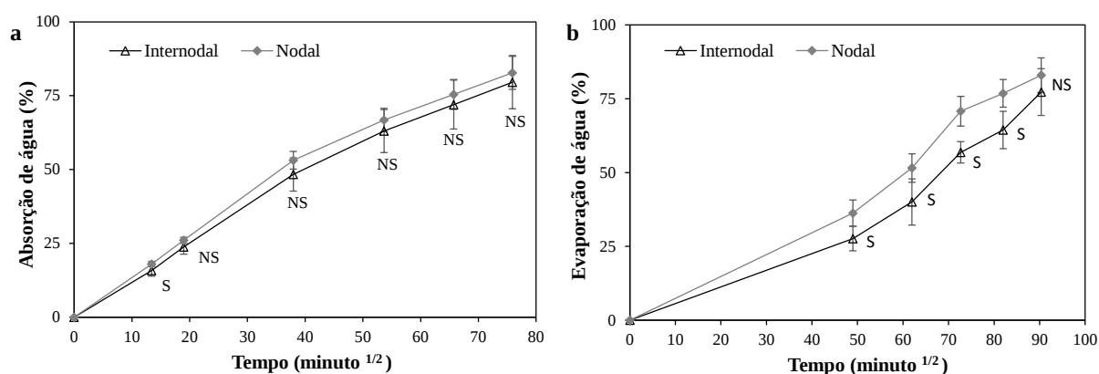
Figura 4.7 - Diagramas de absorção e evaporação de água do bambu. (a) absorção; (b) evaporação. n=5 . (S) variância significativa; (NS) variância não significativa. P < 0,05 . Teste t – Student e Wilcoxon.
