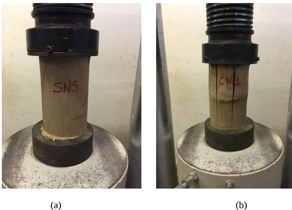
Figura 4.14 - Ruptura à compressão bambu. (a) Sem nó; (b) Com nó.
