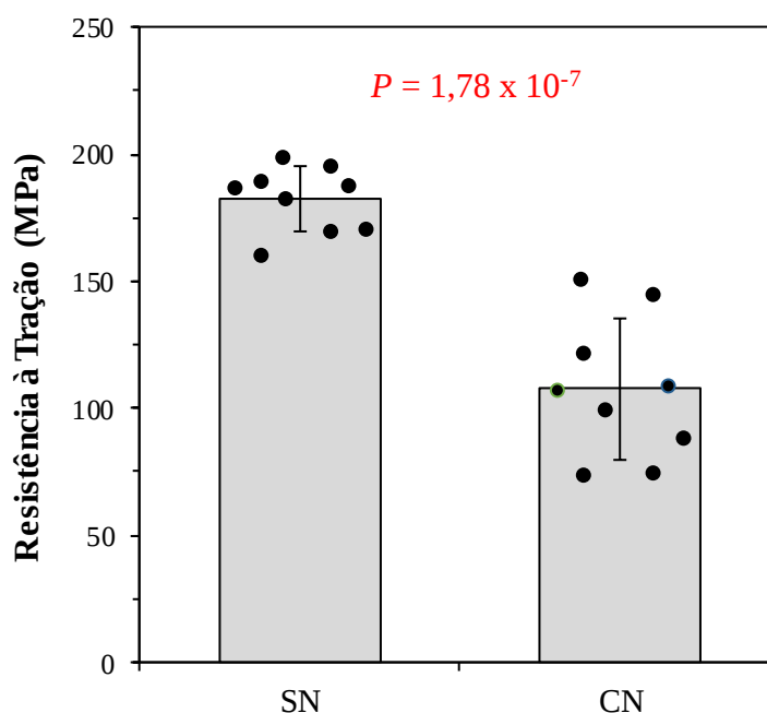
Figura 4.9 - Resultados do ensaio de tração do bambu Dendrocalamus giganteus . (SN) sem nó; (CN) com nó; n=9, variância significativa quando P < 0,05 . Teste t – Student.
