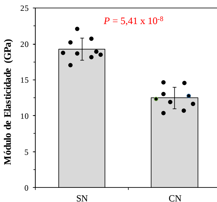
Figura 4.12 - Resultados de módulo de elasticidade do bambu Dendrocalamus giganteus . (SN) sem nó; (CN) com nó; n=9, variância significativa quando P < 0,05 . Teste t – Student.
