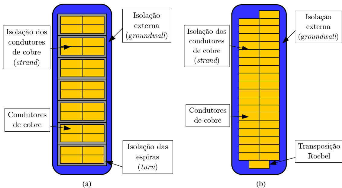
Figura 7 – Tipos de isolamento em (a) bobinas de múltiplas espiras e em (b) barras Roebel. Adaptada de [26].
