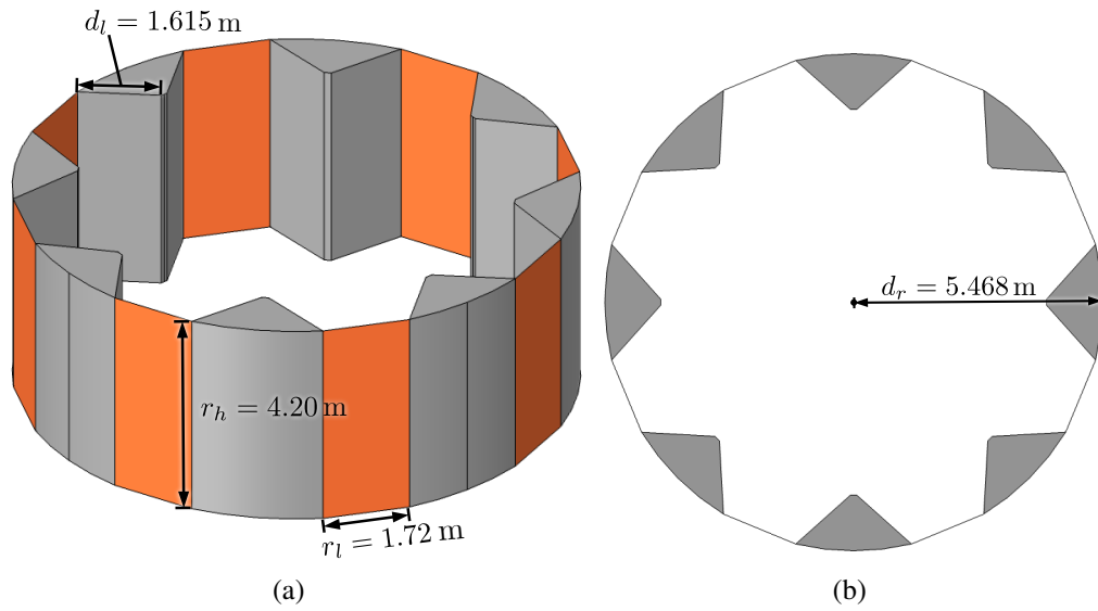
Figura 12 – Direcionadores de ar e radiador do hidrogerador: (a) vista em perspectiva e (b) vista superior. As dimensões d_l , r_l , r_h e d_r são fornecidas.
