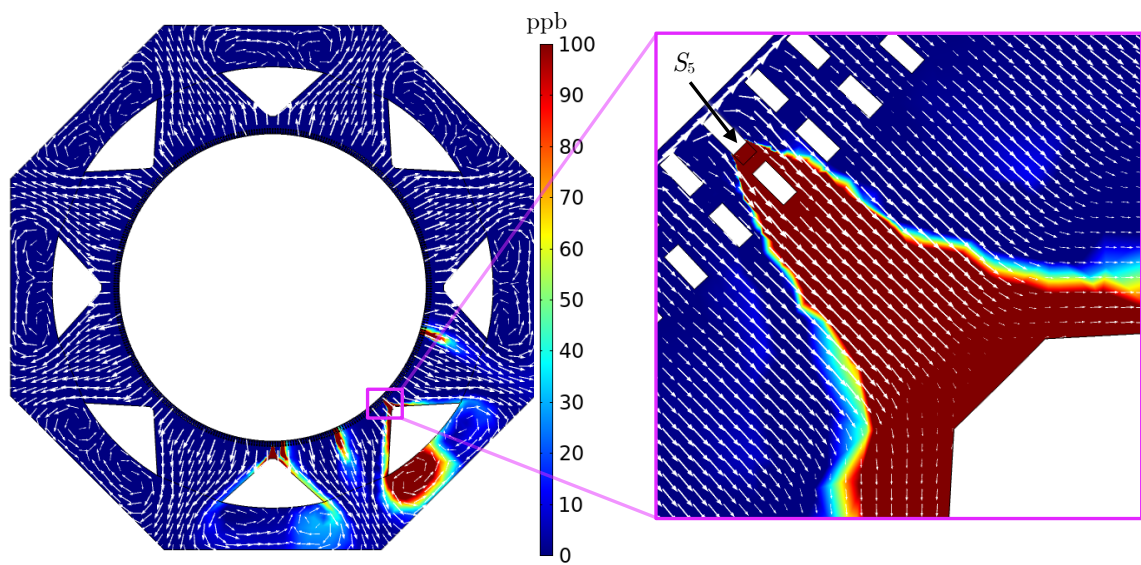
Figura 29 – Distribuição de ozônio (ppb) e campo de velocidade no plano horizontal perpendicular à fonte S_5 (simulação D, z = 2, 070 m).
