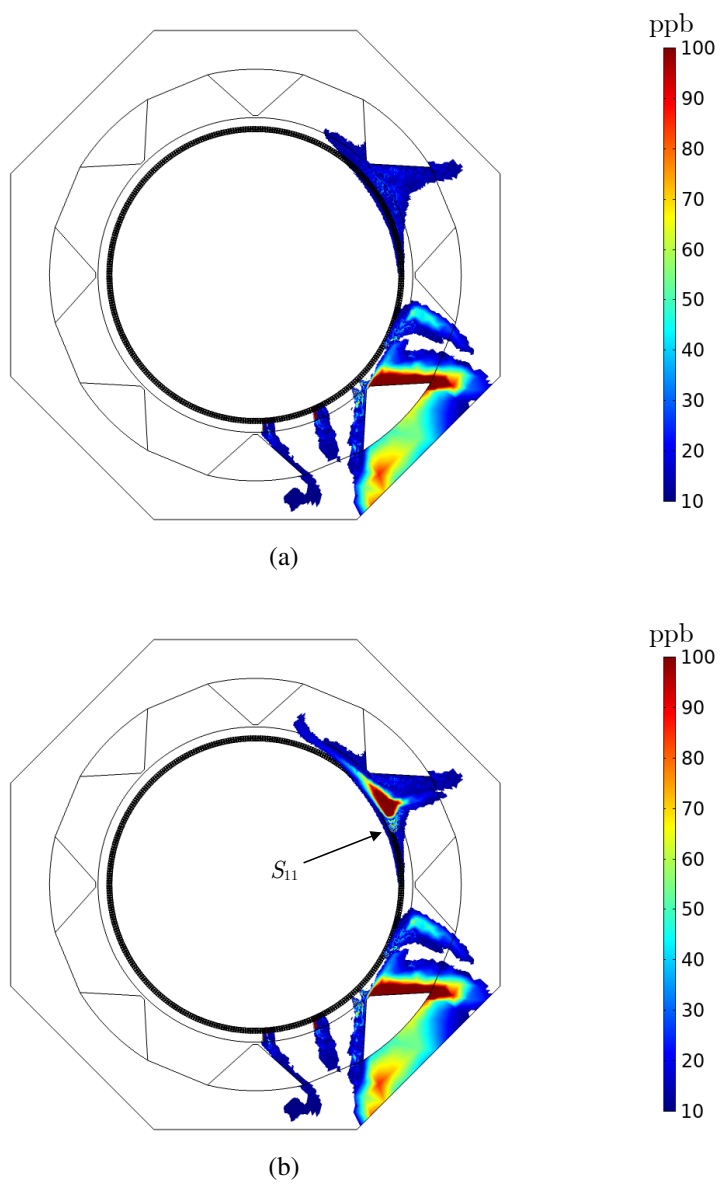
Figura 24 – Visão superior da concentração de ozônio (ppb) no modelo numérico do hidrogerador nas simulações: (a) A e (b) B (fonte S_{11} adicionalmente ativada).
