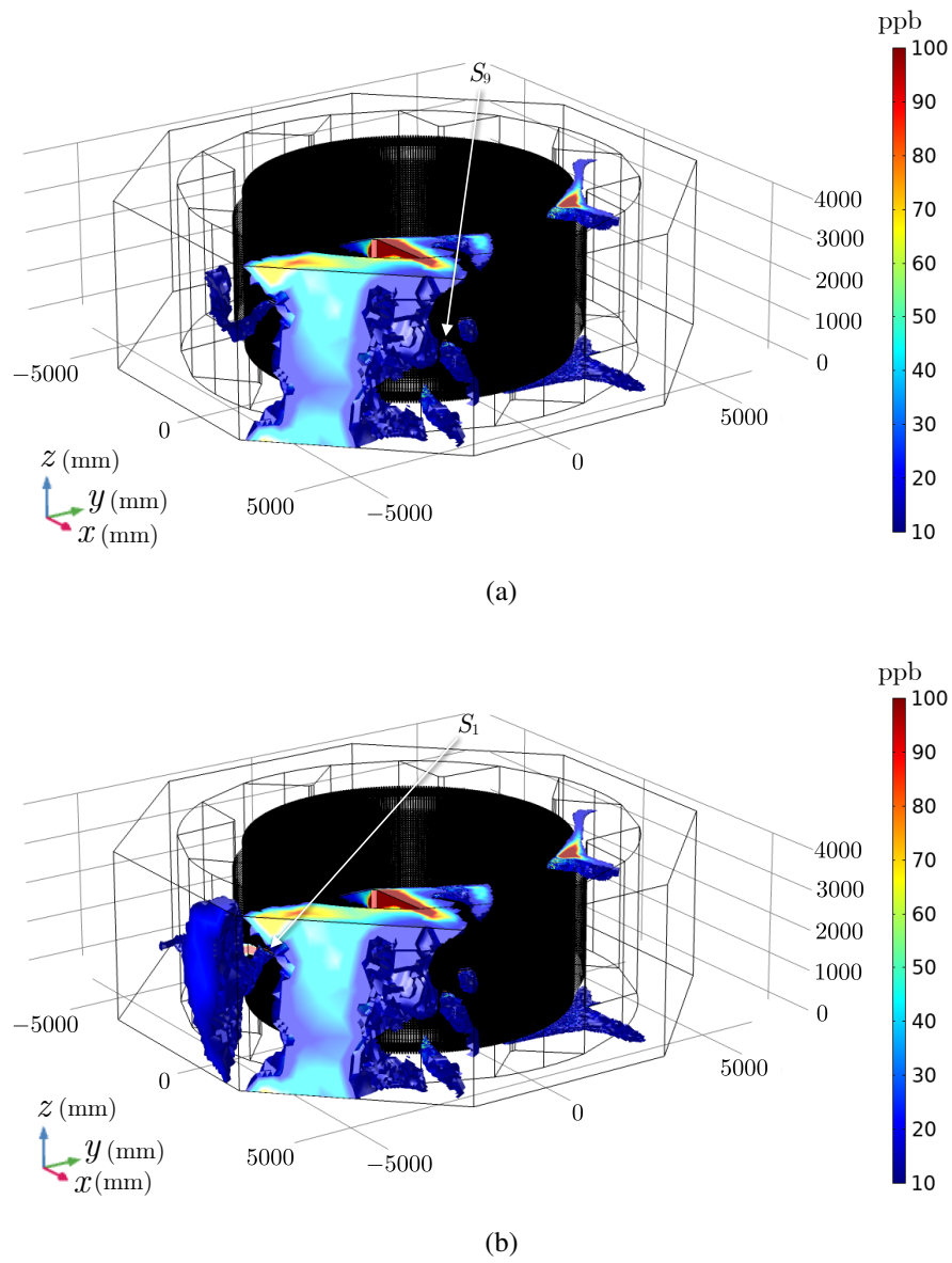
Figura 23 – Visão geral da concentração de ozônio (ppb) no modelo numérico do hidrogerador nas simulações: (a) C (fonte S_9 adicionalmente ativada) e (b) D (fonte S_1 adicionalmente ativada).
