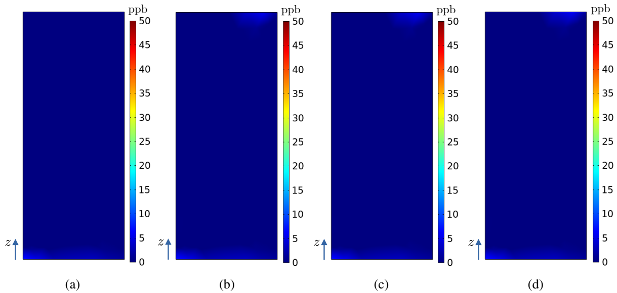
Figura 35 – Concentrações de ozônio (ppb) na superfície do radiador R_5 no modelo numérico do hidrogerador para as simulações: (a) A, (b) B, (c) C e (d) D.
