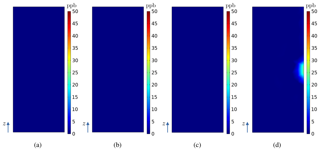
Figura 31 – Concentrações de ozônio (ppb) na superfície do radiador R_1 no modelo numérico do hidrogerador para as simulações (a) A, (b) B, (c) C e (d) D.
