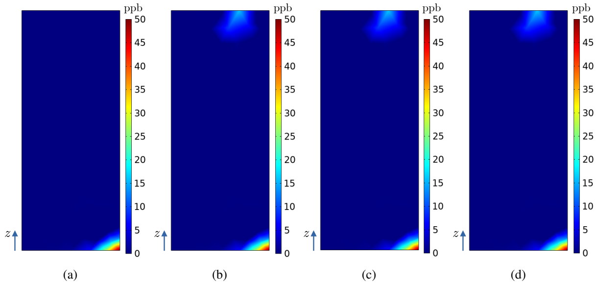
Figura 34 – Concentrações de ozônio (ppb) na superfície do radiador R_4 no modelo numérico do hidrogerador para as simulações: (a) A, (b) B, (c) C e (d) D.
