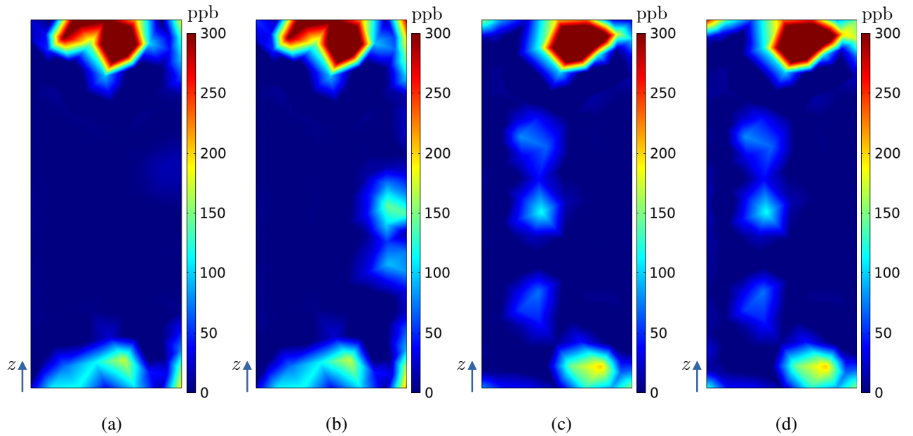
Figura 43 – Concentração de ozônio (ppb) nas superfícies dos radiadores R_5 e R_6 no modelo numérico do hidrogerador: (a) R_5 (simulação E), (b) R_5 (simulação F), (c) R_6 (simulação E) e (d) R_6 (simulação F).
