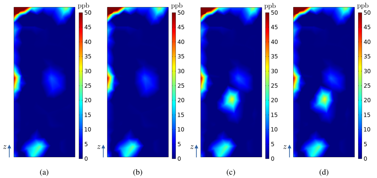
Figura 33 – Concentrações de ozônio (ppb) na superfície do radiador R_3 no modelo numérico do hidrogerador para as simulações: (a) A, (b) B, (c) C e (d) D.
