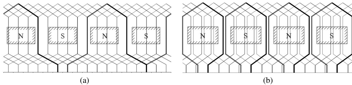
Figura 4 – Ligação das bobinas de acordo com o tipo de barras Roebel: (a) ondulada e (b) imbricada. Reproduzida de [26].
