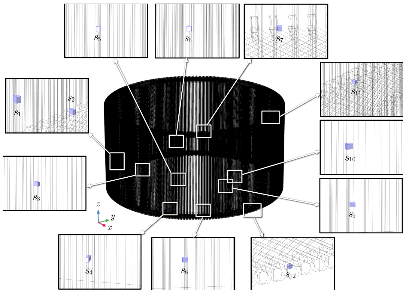
Figura 13 – Posicionamento das fontes (e seus rótulos) nas barras estatóricas do hidrogerador.
