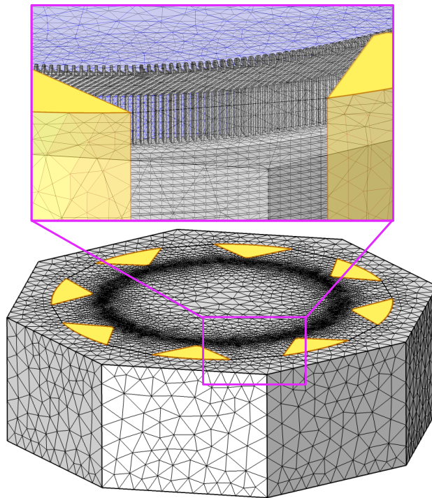
Figura 14 – Visão geral da malha de elementos finitos concebida para representar a estrutura do hidrogerador. As regiões amareladas são os direcionadores de ar.
