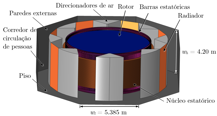
Figura 9 – Visão geral do modelo de elementos finitos do hidrogerador: rotulação das partes estruturais. A altura w_h e largura w_l da parede são fornecidas.
