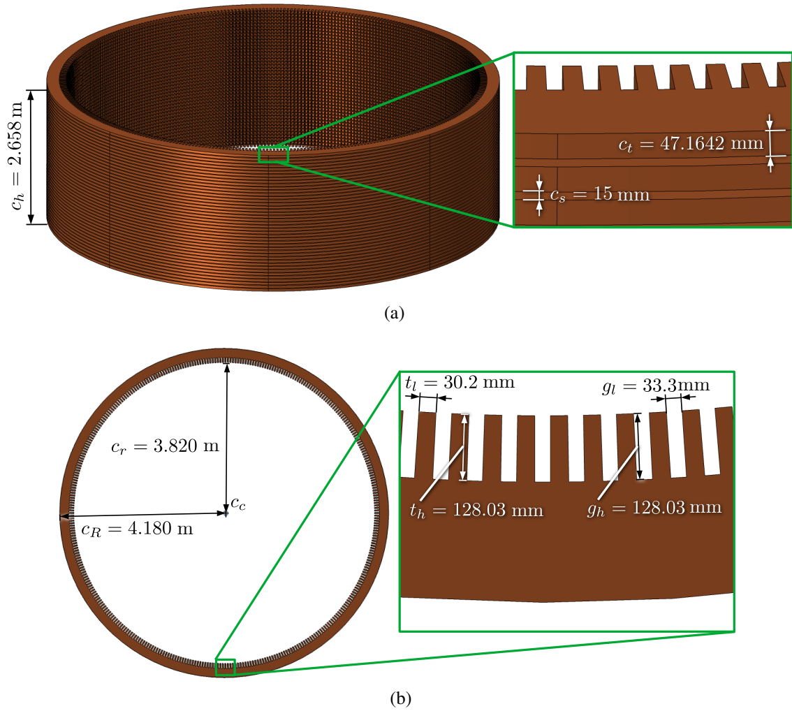
Figura 11 – Núcleo estático do hidrogerador e suas dimensões: (a) vista em perspectiva e (b) vista superior. As dimensões c_h , c_t , c_s , c_r , c_R , t_l , g_l , t_h e g_h são fornecidas.
