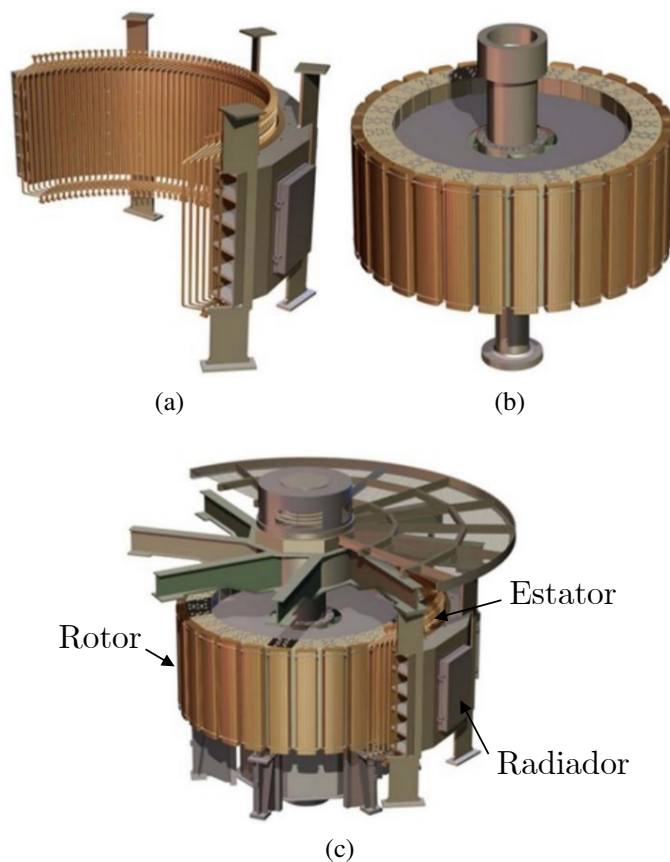
Figura 1 – Principais estruturas elétricas de um hidrogerador: (a) parte do estator, (b) rotor e (c) estrutura contendo estator e rotor. Adaptada de [25].
