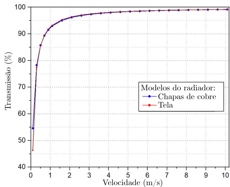
Figura 16 – Transmissões de ozônio através de modelos numéricos de radiadores em função da velocidade do ar: modelos de chapas de cobre e tela.
