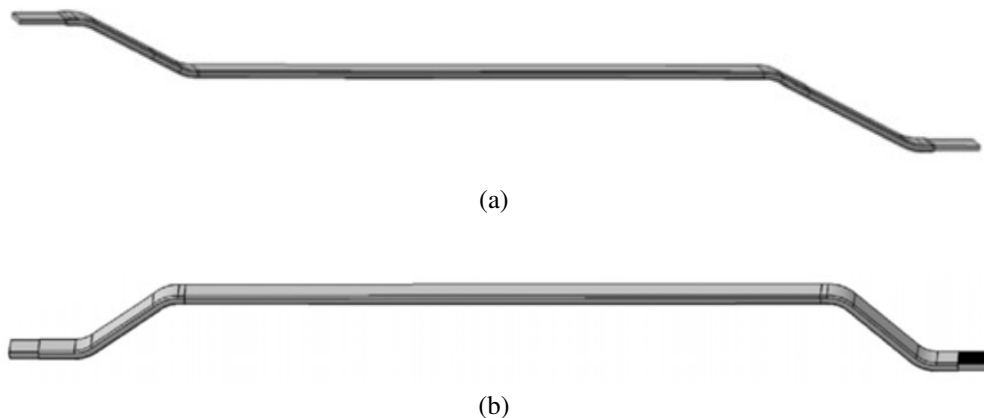
Figura 3 – Modelos de barras Roebel: (a) barra do tipo ondulada e (b) barra do tipo imbricada. Adaptada de [26].
