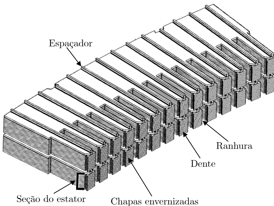
Figura 2 – Estrutura do núcleo estatórico. Adaptada de [27].
