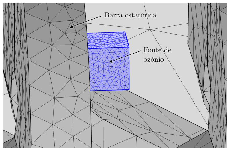
Figura 15 – Parte da malha computacional concebida para representar as fontes de ozônio (destacadas em azul) e as barras estatóricas.
