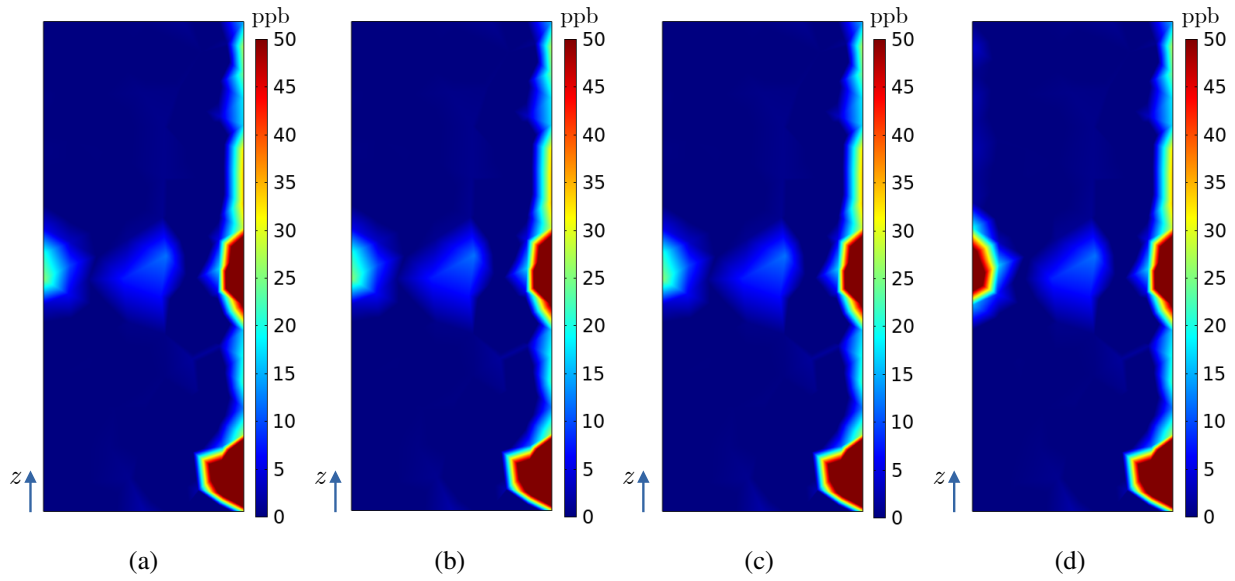
Figura 32 – Concentrações de ozônio (ppb) na superfície do radiador R_2 no modelo numérico do hidrogerador para as simulações: (a) A, (b) B, (c) C e (d) D.
