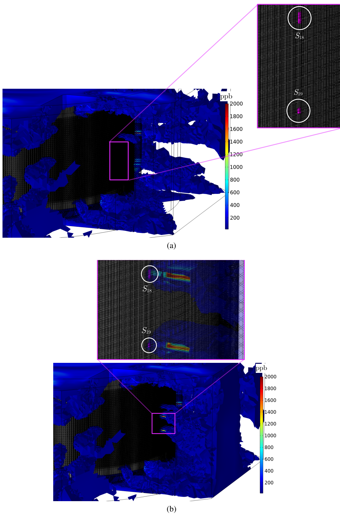
Figura 37 – Influência localizada na região das fontes S_{18} e S_{19} na simulação: (a) E e (b) F.
