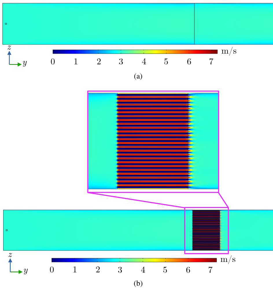
Figura 18 – Magnitude do campo de velocidade (m/s) no plano yz nas simulações de referência: (a) modelo de tela do radiador e (b) representação realista em cobre do radiador.
