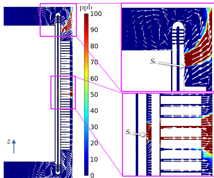
Figura 27 – Distribuição de ozônio (ppb) e campo de velocidade no plano vertical perpendicular às fontes S_5 e S_6 (simulação D, \phi = 315^\circ ).
