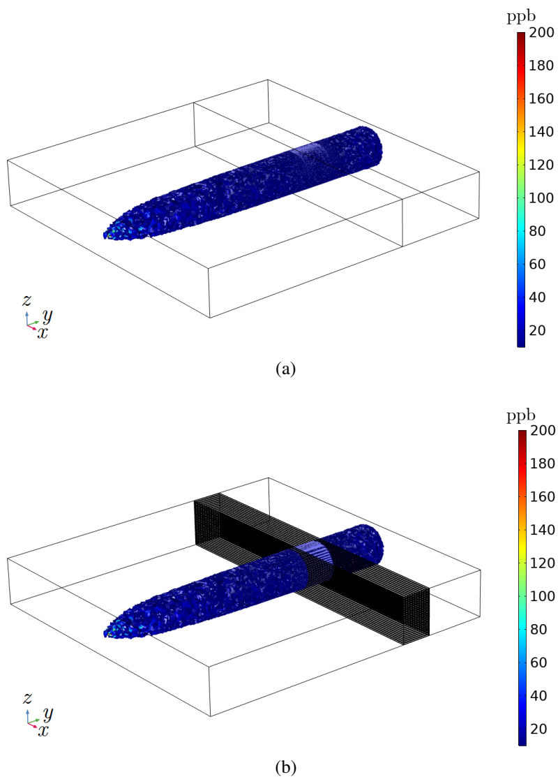
Figura 17 – Vistas em perspectiva das distribuições de concentração de ozônio (ppb) em simulações de referência: (a) modelo de tela do radiador e (b) representação realista em cobre do radiador.
