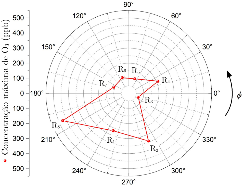
Figura 45 – Concentrações máximas de ozônio nos radiadores em função de \phi (modelo numérico).
