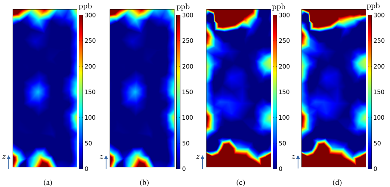
Figura 44 – Concentração de ozônio (ppb) nas superfícies dos radiadores R_7 e R_8 no modelo numérico do hidrogerador: (a) R_7 (simulação E), (b) R_7 (simulação F), (c) R_8 (simulação E) e (d) R_8 (simulação F).
