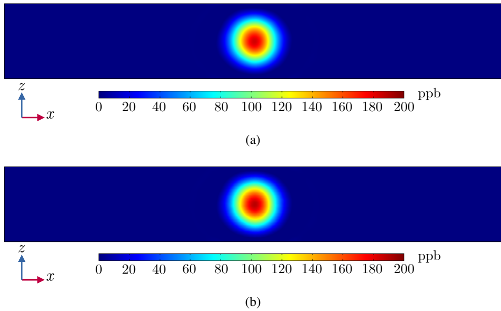
Figura 20 – Concentrações de ozônio (ppb) no plano xz nas simulações de referência: (a) modelo de tela do radiador e (b) representação realista em cobre do radiador.
