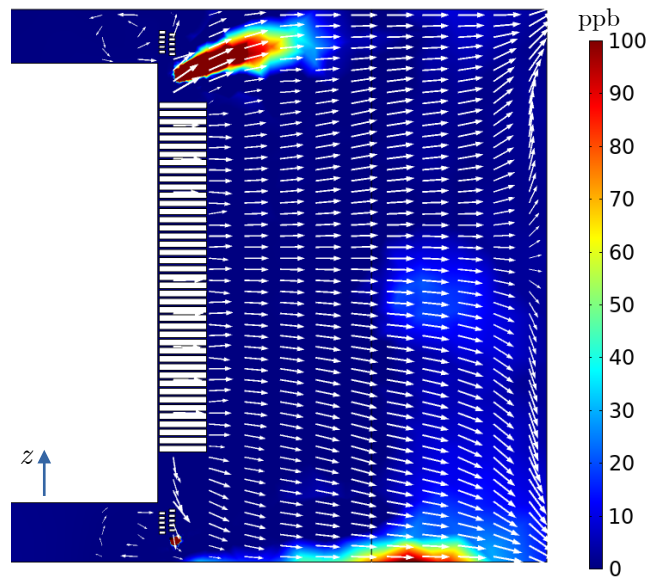
Figura 28 – Distribuição de ozônio (ppb) e campo de velocidade no plano vertical perpendicular ao radiador R_3 (simulação D, \phi = 337, 5^\circ ).
