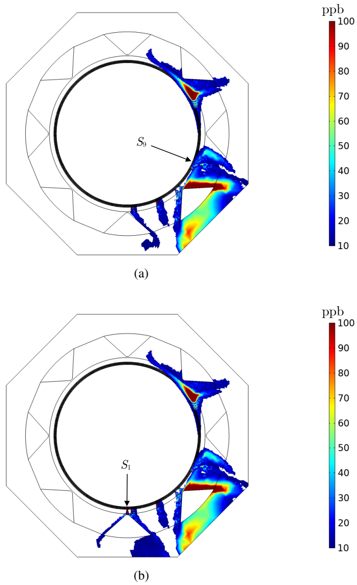
Figura 25 – Visão superior da concentração de ozônio (ppb) no modelo numérico do hidrogerador nas simulações: (a) C ( S_9 adicionalmente ativada) e (b) D ( S_1 adicionalmente ativada).
