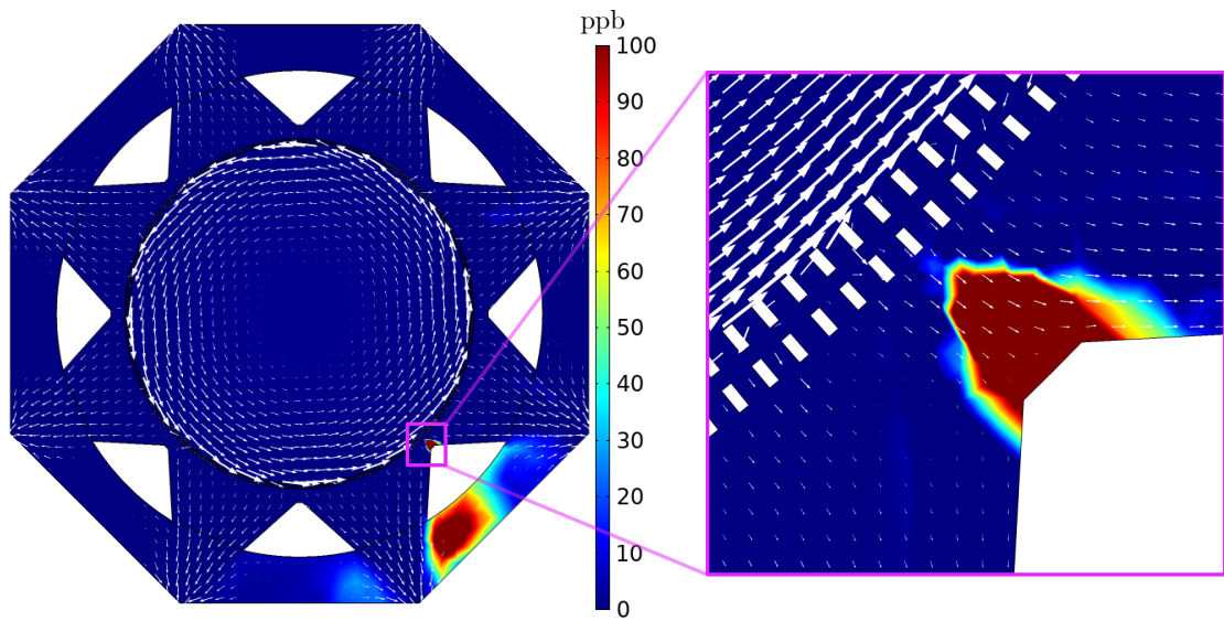
Figura 30 – Distribuição de ozônio (ppb) e campo de velocidade em um plano horizontal na região superior do hidrogerador (simulação D, z = 3,750 m).
