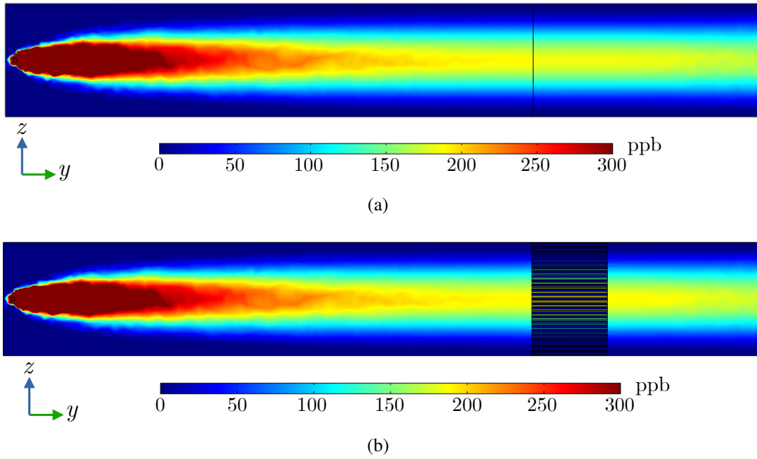
Figura 19 – Concentrações de ozônio (ppb) no plano yz nas simulações de referência: (a) modelo de tela do radiador e (b) representação realista em cobre do radiador.
