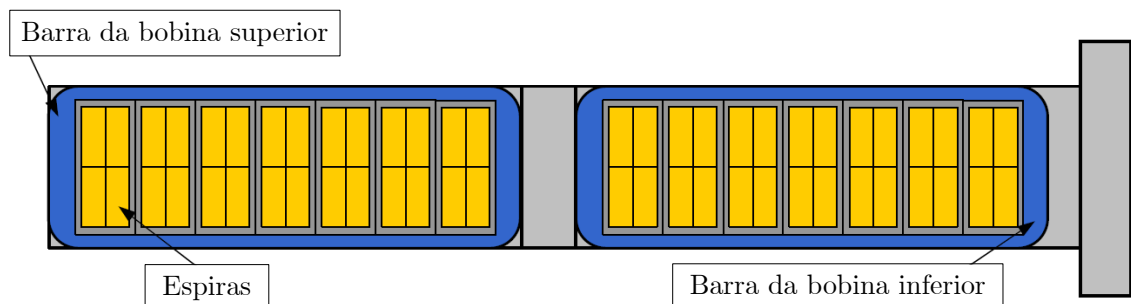
Figura 6 – Corte de uma ranhura com bobina de múltiplas espiras. Adaptada de [28].
