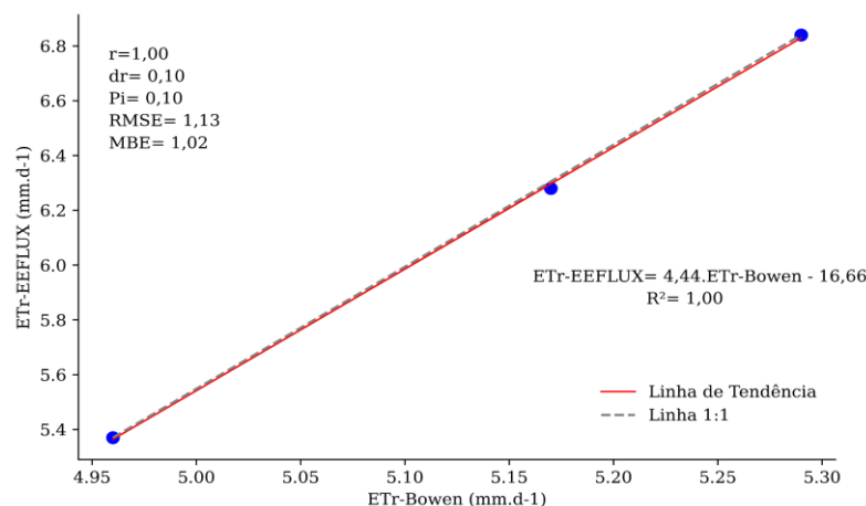
Figura 11 - Dispersão entre a ETr-EEFLUX e a ETr-Bowen ao redor da linha 1:1, coeficientes de correlação ( r ) e concordância ( dr ), índices estatísticos RMSE e MBE e desempenho P_i da cultura da mangueira Tommy Atkins
