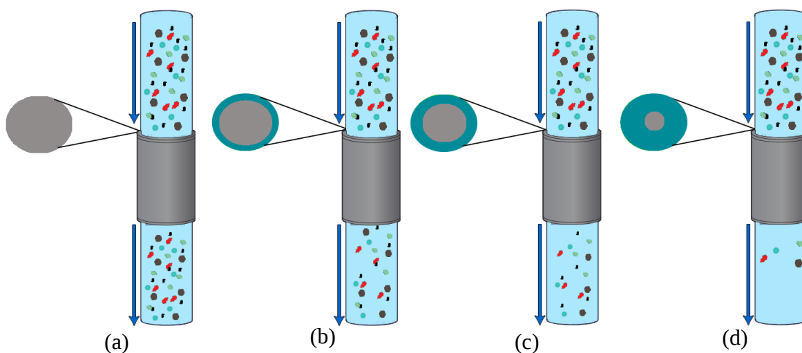
Figura 3: Representação das fases do fouling causado por moléculas orgânicas.
