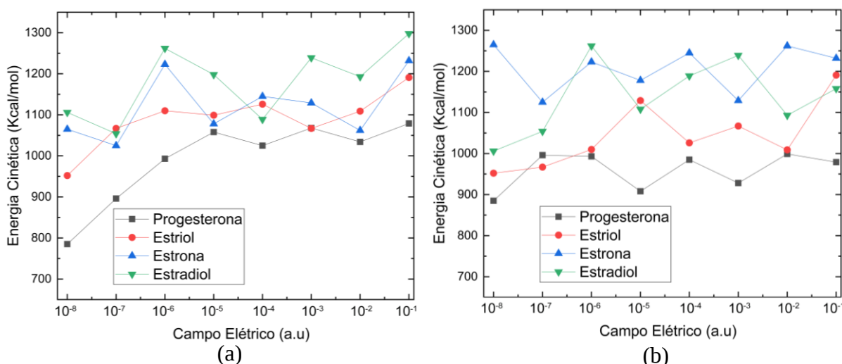
Figura 13: Energia cinética dos hormônios naturais na NF em: a) NTC e b) NTNBN.
