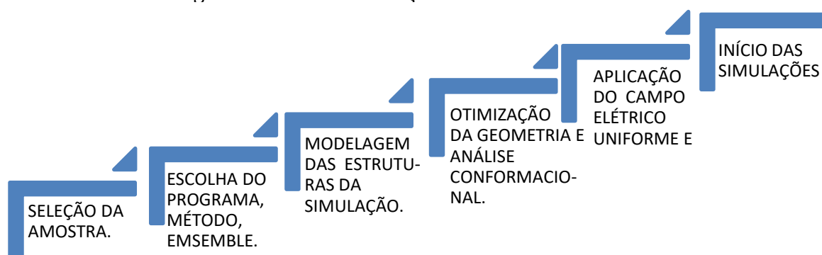
Figura 6: Fases da simulação da DM.
