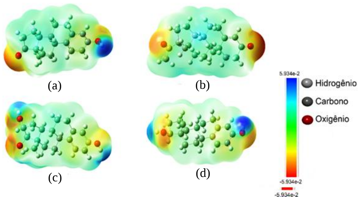
Figura 19: MEP dos hormônios naturais: a) E 1 b) PGR, c) E 3 e d) EE 2 .
