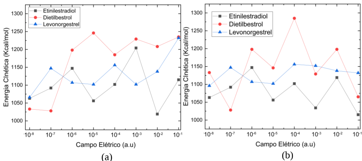
Figura 14: Energia cinética dos hormônios sintéticos da NF em: a) NTC e b) NTN. B.
