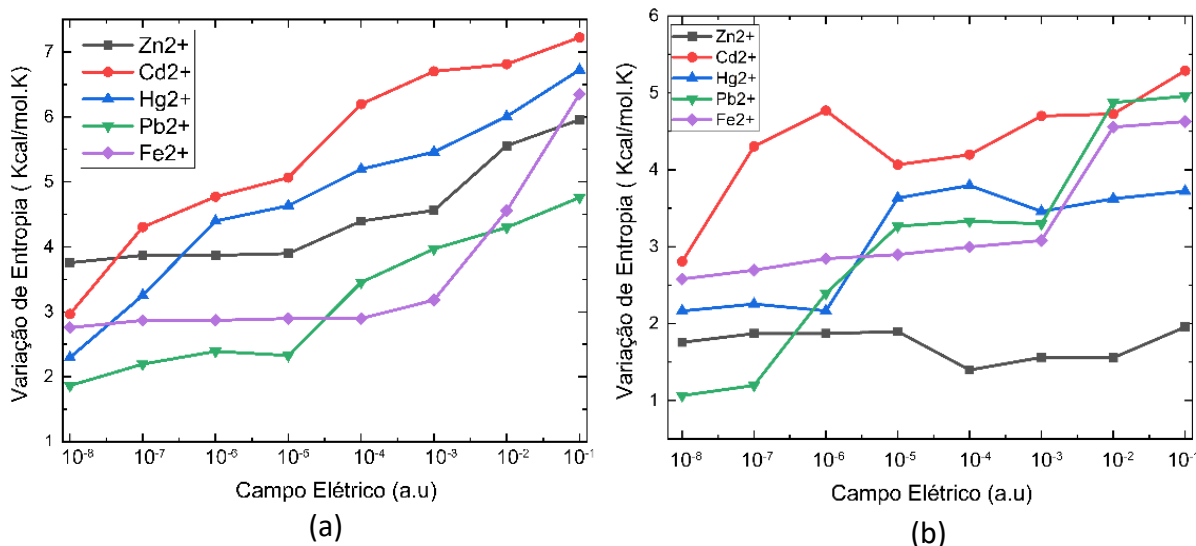
Figura 11: Entropia dos íons de MP na NF em: a) NTC e b) NTNB.
