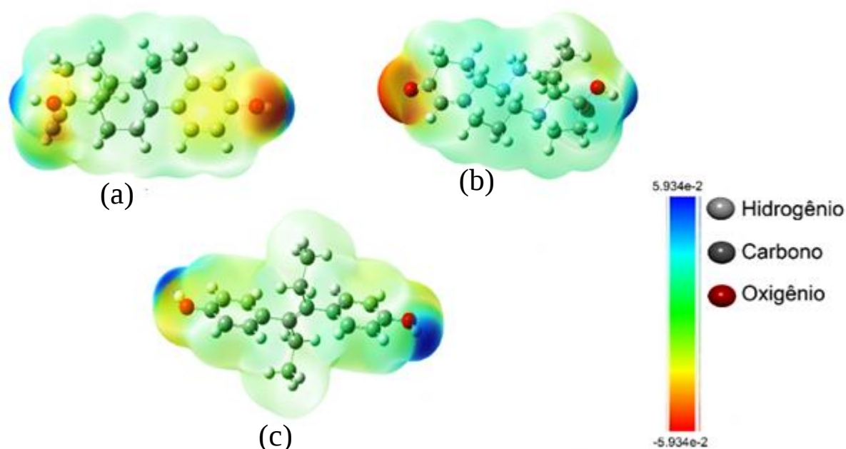
Figura 21: MEP dos hormônios sintéticos: a) EE 2 , b) LNG e c) DES.
