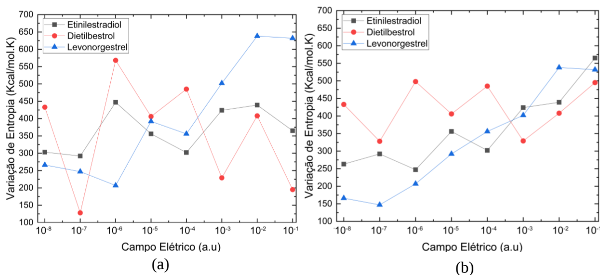
Figura 16: Entropia dos hormônios sintéticos na NF em: a) NTC e b) NTNB.
