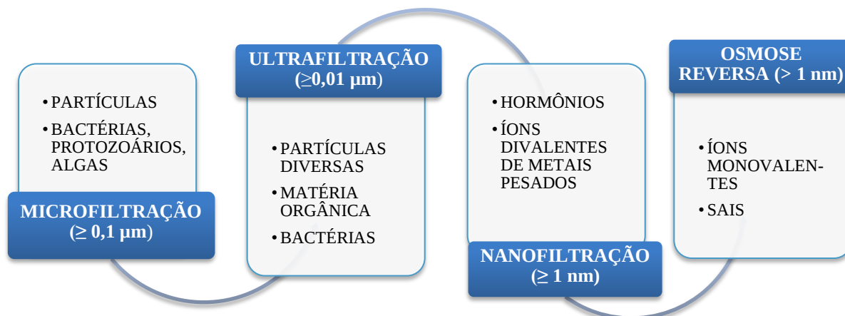
Figura 1: Processos de separação das ETE.
