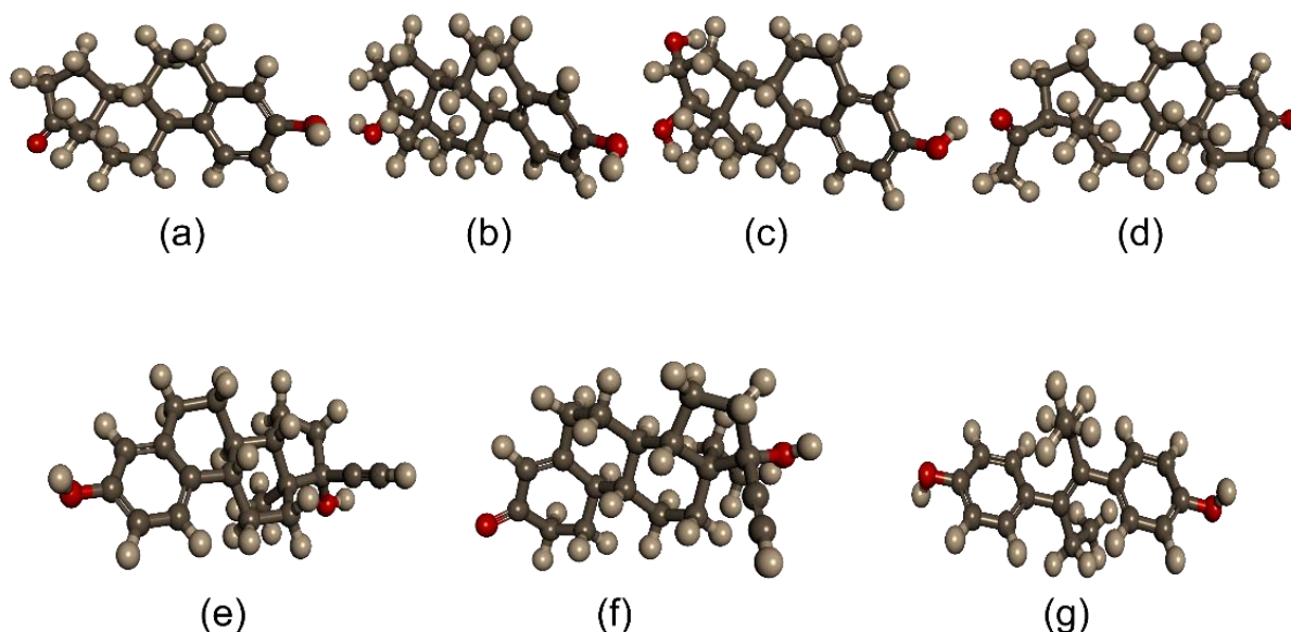
Figura 7: Moléculas de Hormônios: a) E 1 , b) E 2 , c) E 3 ; d) PGR, e) EE 2 , f) LNG e g) DES.
