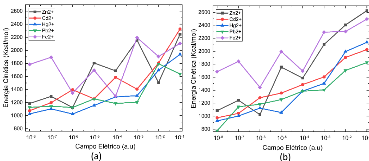
Figura 10: Energia cinética dos íons de MP na NF em: a) NTC e b) NTNb.
