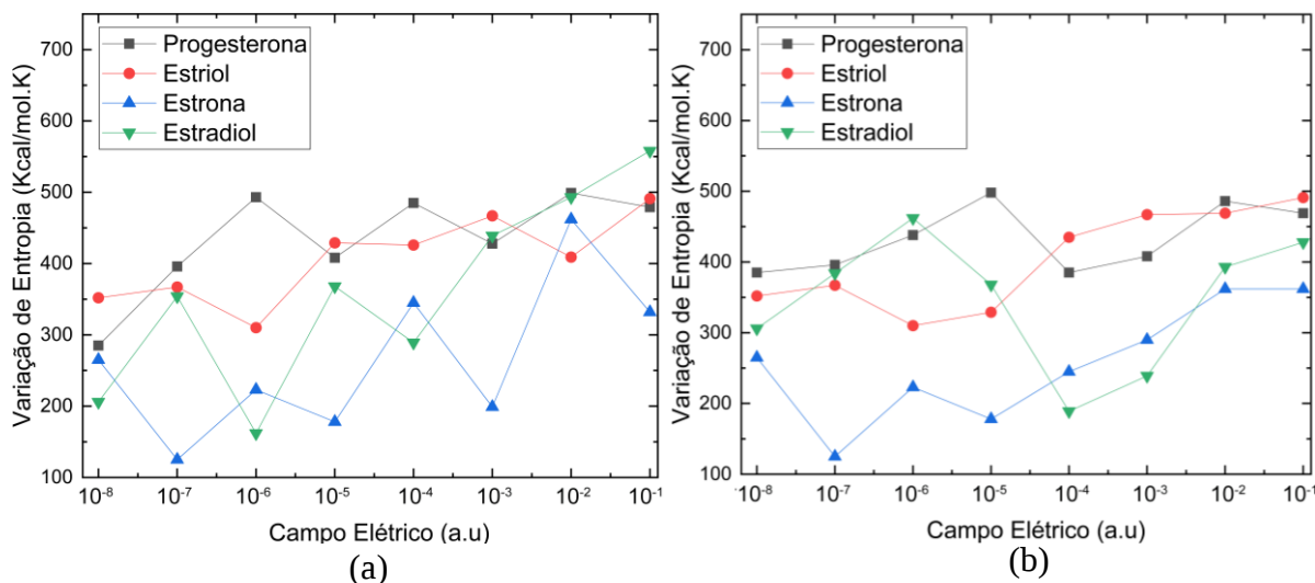
Figura 15: Entropia dos hormônios naturais na NF em: a) NTC e b) NTN. B.
