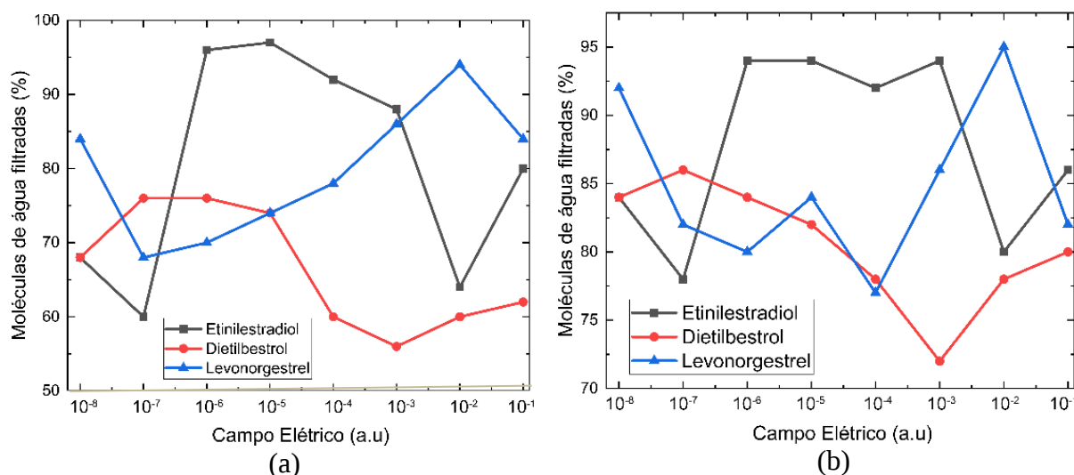
Figura 20: NF de hormônios sintéticos em: a) NTC e b) NTNB.
