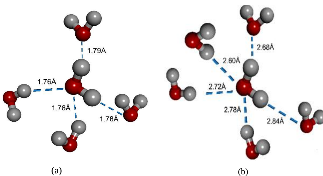
Figura 5: Distância das ligações de hidrogênio: a) na água livre e b) em água confinada sob CEU de 10^{-8} a.u.
