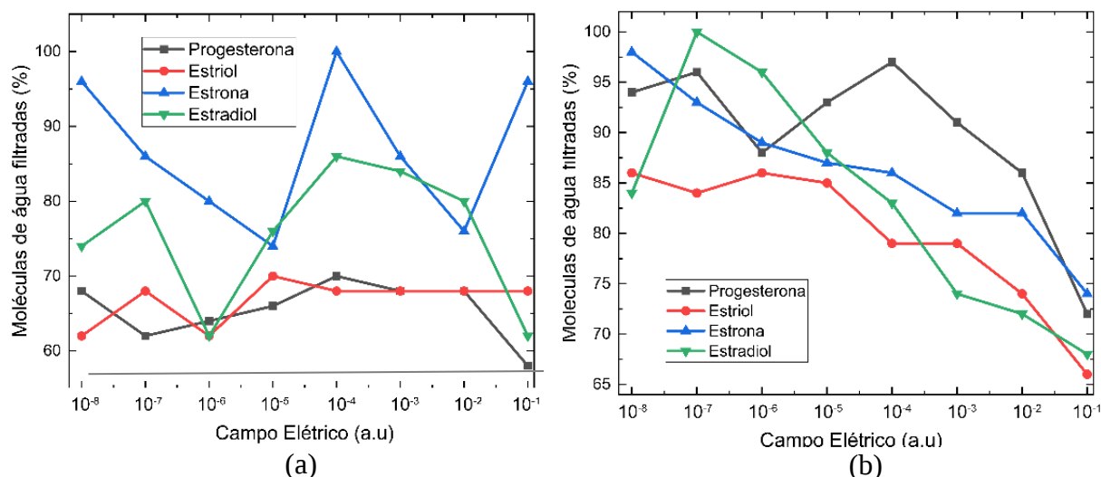
Figura 17: NF de hormônios naturais em: a) NTC e b) NTNB.
