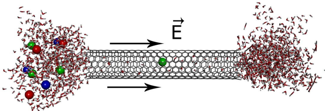
Figura 9: CEU intensifica e direciona a cinética da água no sentido da NF.
