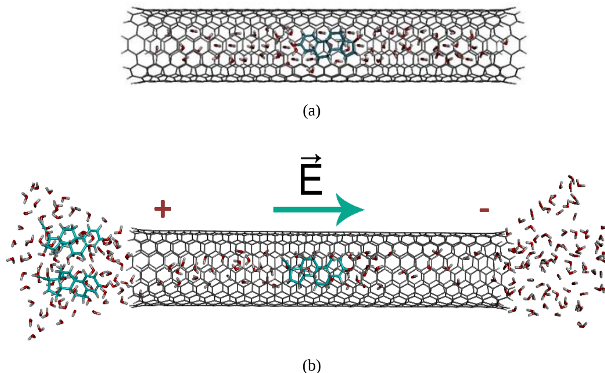
Figura 8: Simulação da DM: a) otimização de geometria e b) aplicação do CEU no NT.
