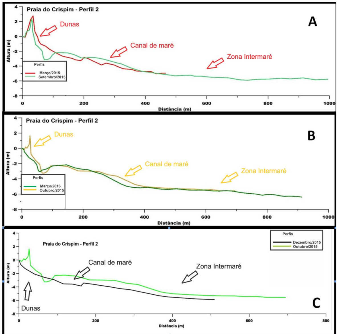
Figura 36- Perfis de comparação por pares dos meses de Março/2015 a Dezembro/2015 para o Perfil 2 na praia do Crispim.
