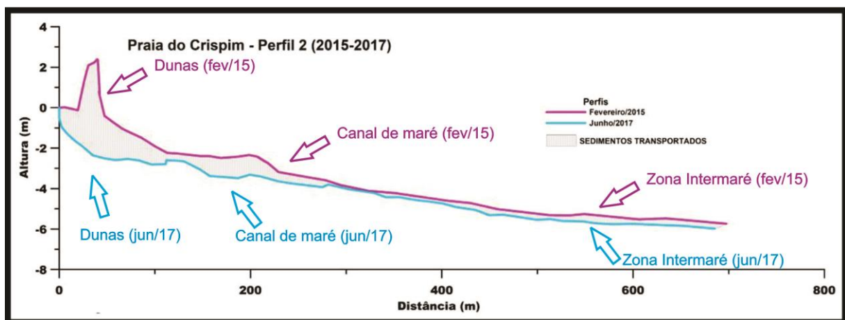
Figura 37- Variação dos perfis topográficos total no período de monitoramento (fevereiro/2015 a junho/2017) no Perfil 2 da praia do Crispim.
