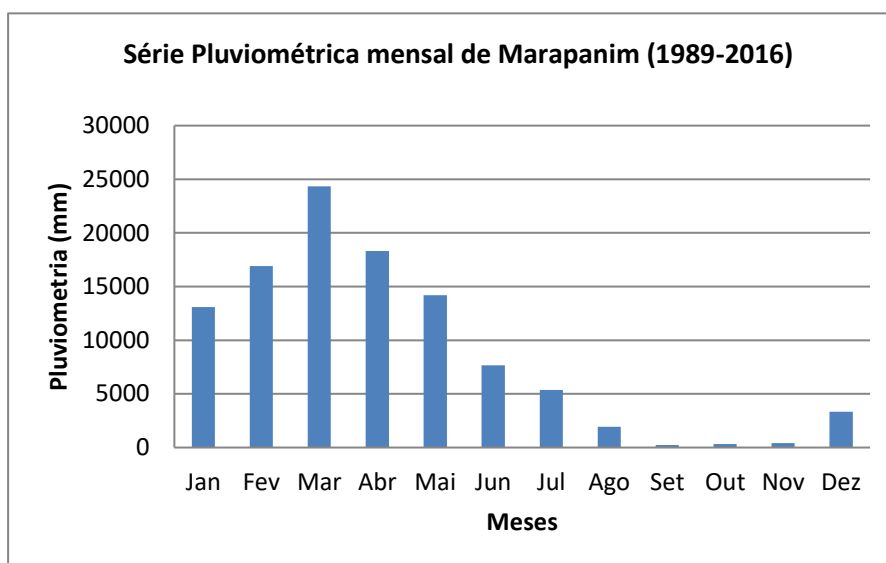
Figura 12- Série histórica da precipitação mensal (1989-2016) no município de Marapanim.
