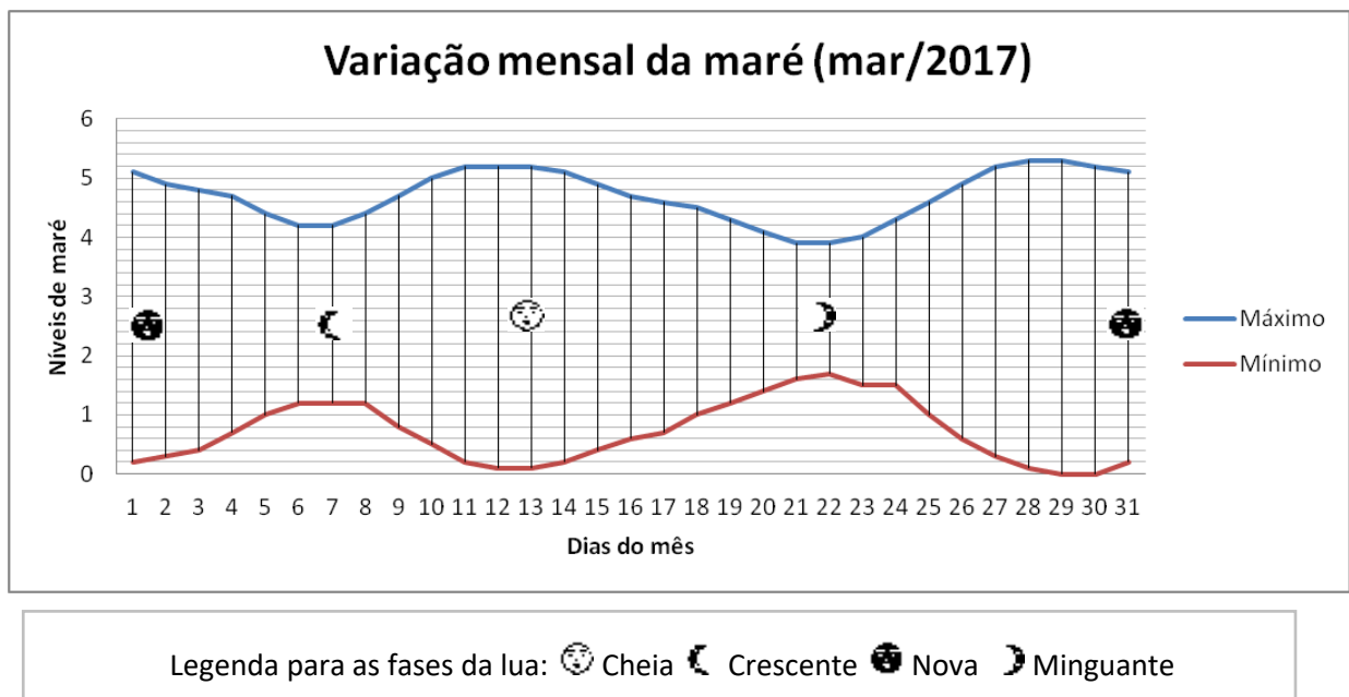
Figura 10- Variação da maré ao longo do mês de março de 2017
