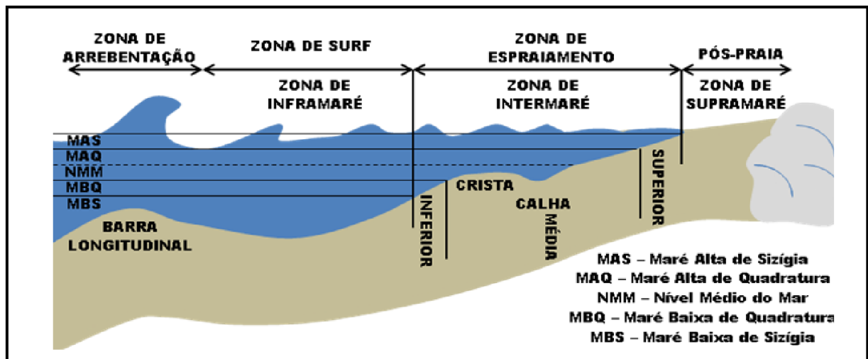
Figura 2- Diagrama do perfil de praias de macromarés segundo a hidrodinâmica e a morfologia.
