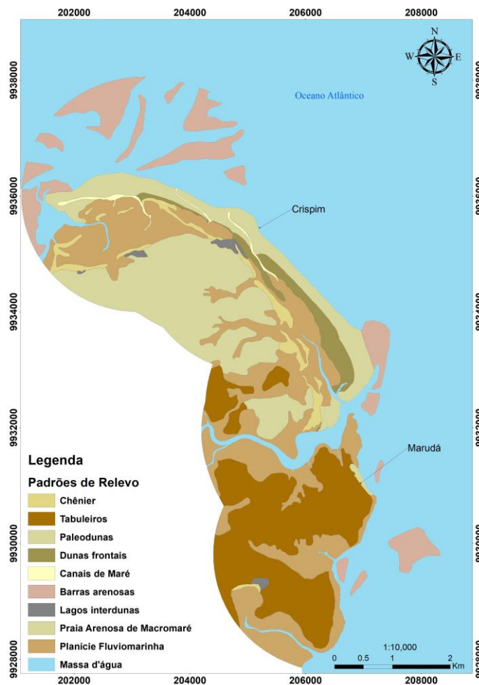
Figura 19- Mapa de unidades geomorfológicas da área de estudo.
