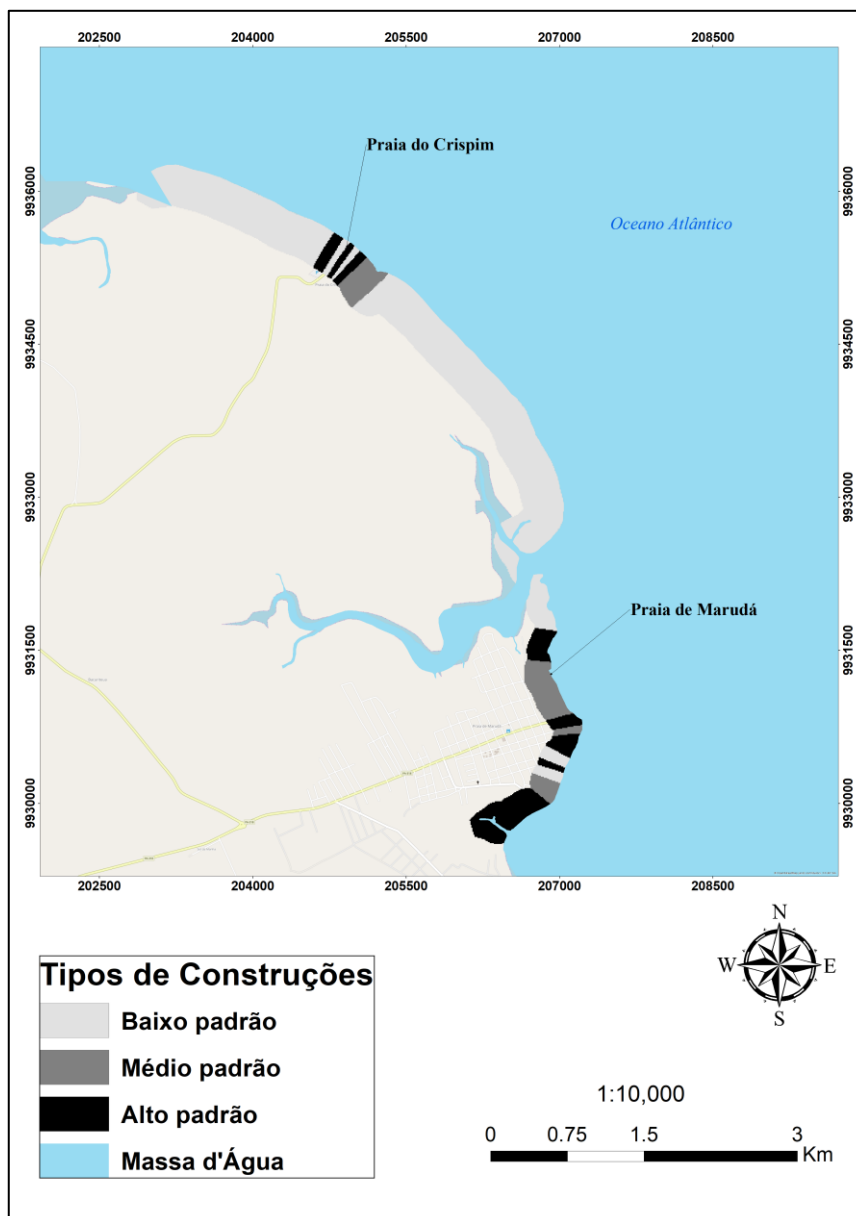
Figura 48- Mapa de tipos de construção com base nos padrões construtivos encontrados na praia do Crispim e Marudá.
