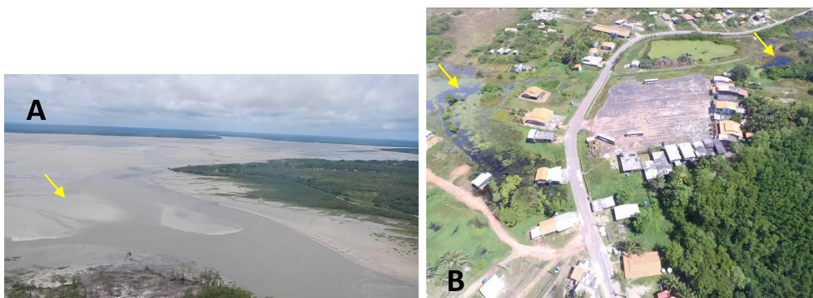
Figura 22- (A) Barras arenosas na foz de rio entre as praias do Crispim e Marudá. (B) Lagos interdunas próximos à comunidade do Crispim.
