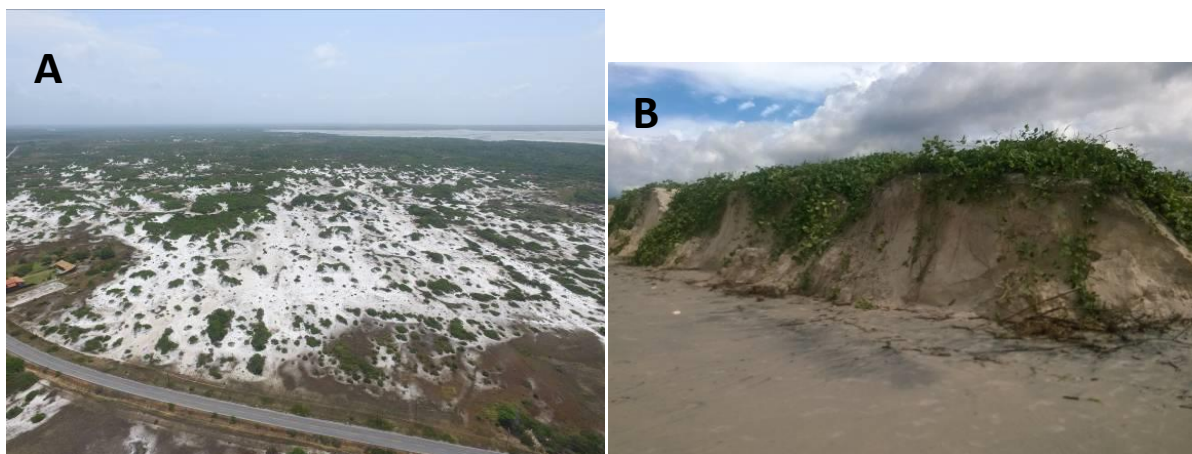
Figura 21- (A) Paleodunas recortada por estrada de acesso à praia do Crispim. (B) Dunas frontais verticalizadas existentes na região central da praia do Crispim em 2015.
