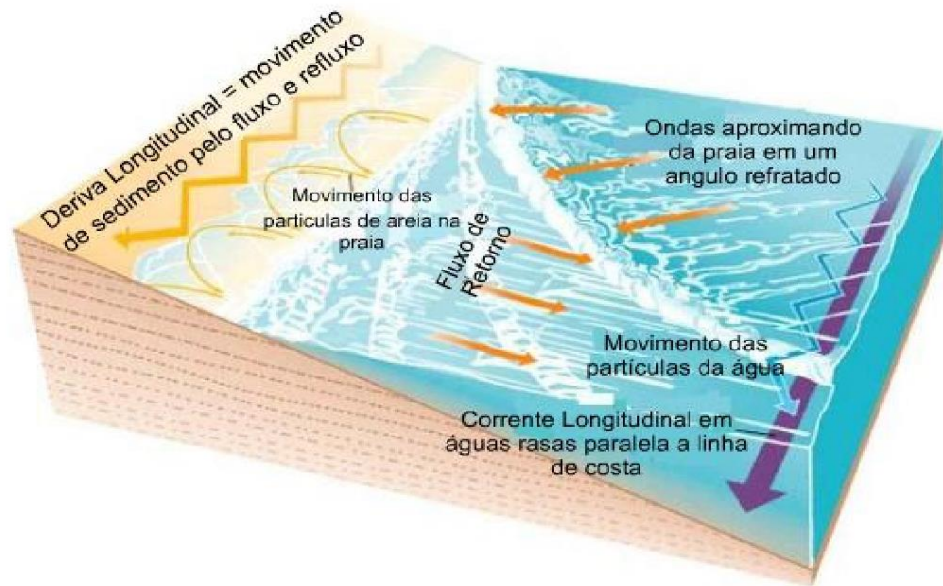
Figura 3- Processos de deriva sedimentar na região costeira.
